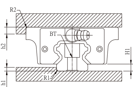
圖2. SR安裝部位(mm)
